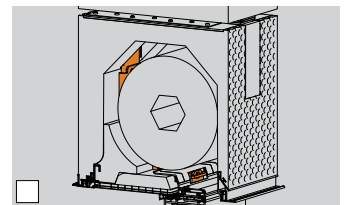
Blendrahmenstabilisierung für zusätzliche Stabilität bei breiten Fenstern
