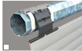
Fester Wellenverbinder zur Einbruchhemmung (nur bei Profil ALUMINO und Motorbedienung).
